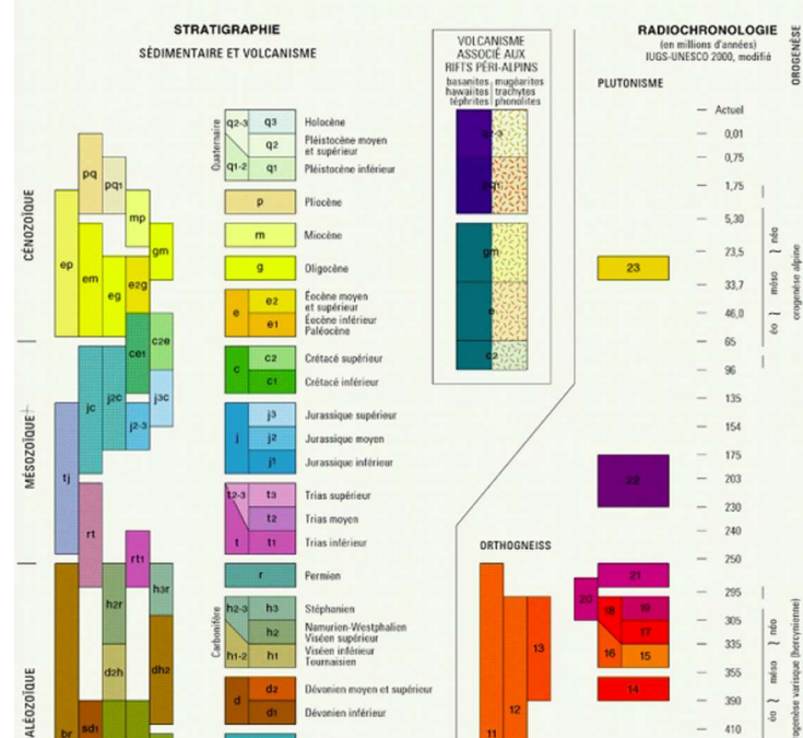
Figure 5 : Extrait de la carte géologique à 1/250 000, feuille Lyon (BRGM)
