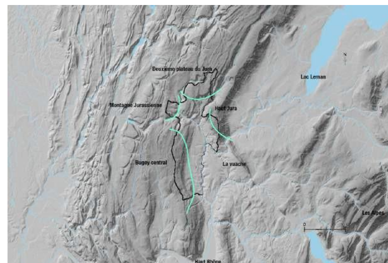
Le relief du territoire (Source : Géoportail ; EAU PROSCOT)
