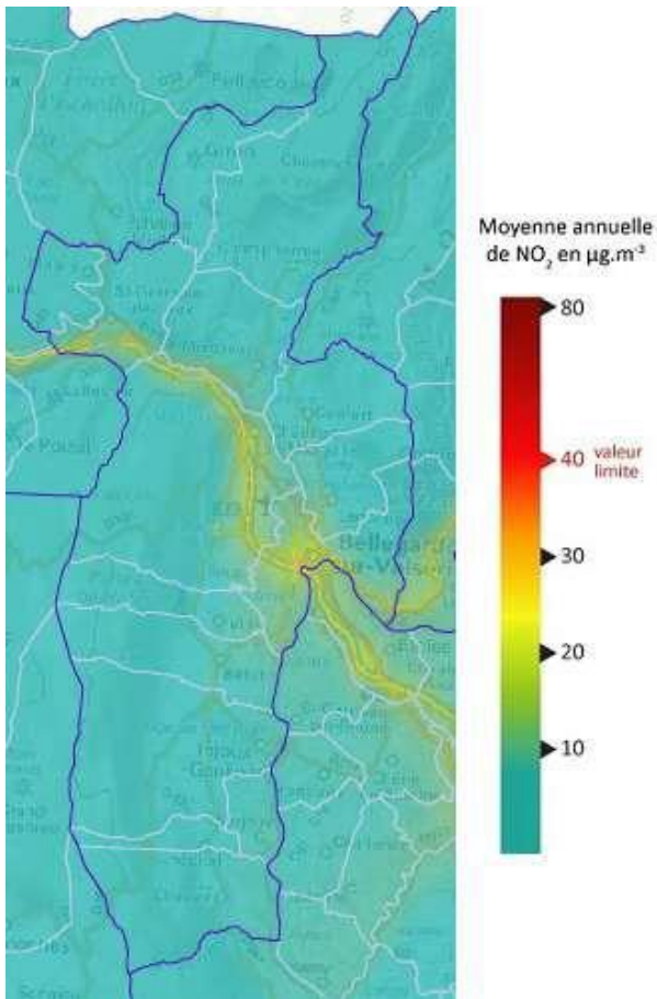
Moyenne annuelle de NO2 sur le territoire du Pays Bellegardien, en 2015 (Source : air-RhôneAlpes)
